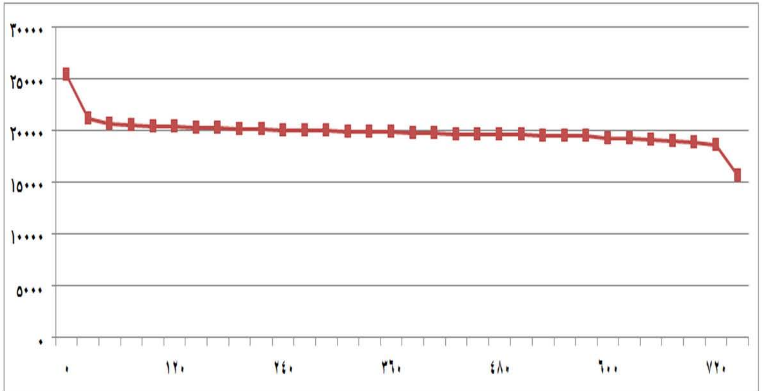
شكل (٨) المنحنى الشهري لفترة الحمل أبريل ٢٠١٧
