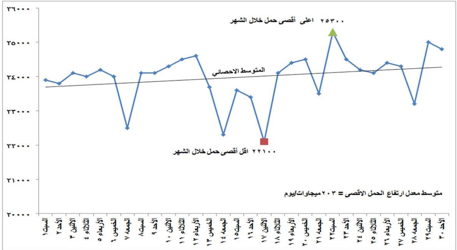
شكل (١) تطور الحمل الاقصى اليومي خلال شهر أبريل ٢٠١٧
