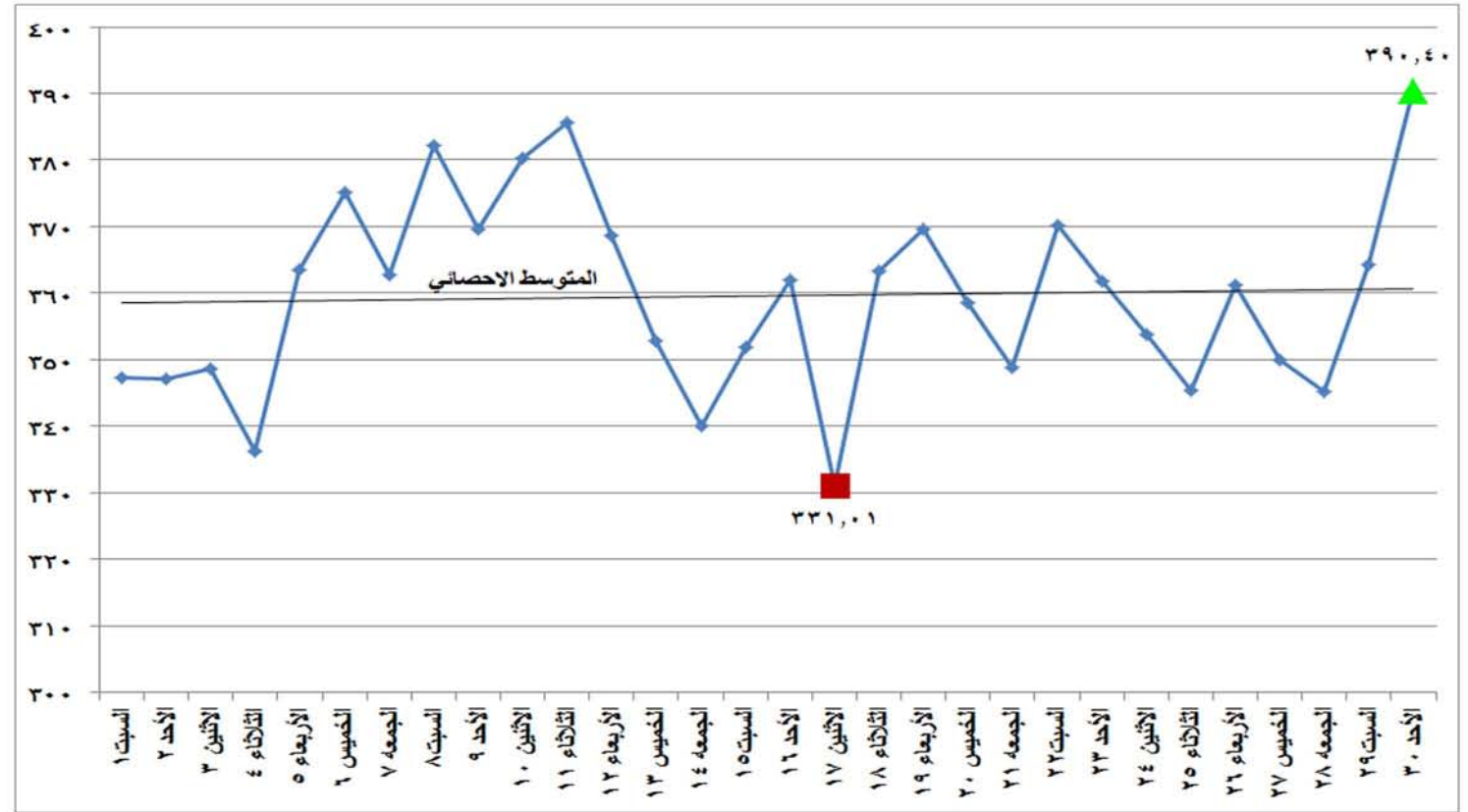
شكل (١٧) الطاقة الكهربائية المنتجة من الغاز الطبيعي خلال شهر أبريل ٢٠١٧
