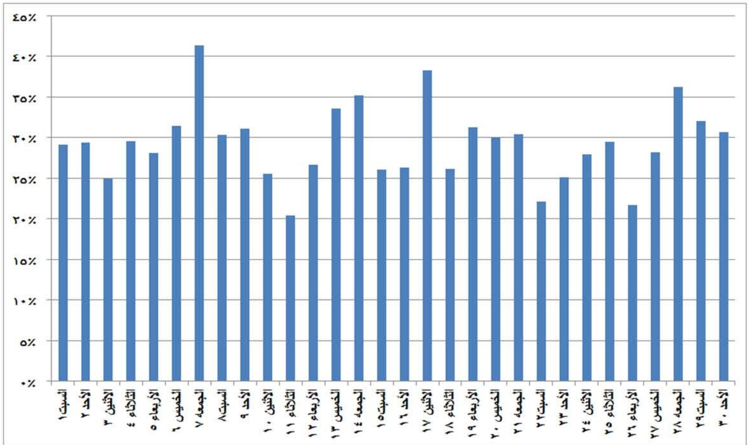
شكل (٢٨) نسب الفائض للحمل الاقصى المسجل يوميا خلال شهر أبريل ٢٠١٧
