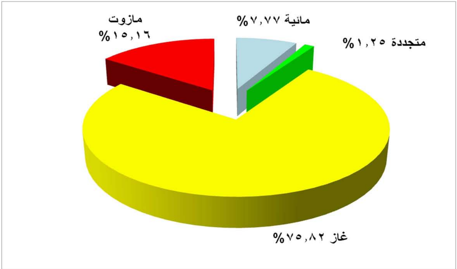
شكل (١٣) متوسط نسب مشاركة مصادر الطاقة الاولية في انتاج الكهرباء خلال شهر أبريل ٢٠١٧
