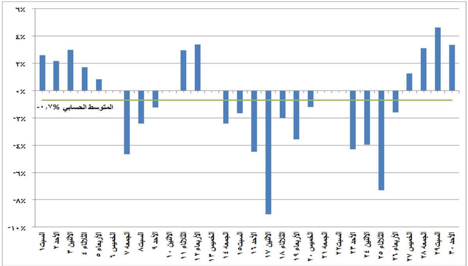
شكل (٩) النسب المئوية للتغير في الحمل الأقصى خلال شهر أبريل ٢٠١٧ مقارنة باليوم المماثل من العام الماضي
