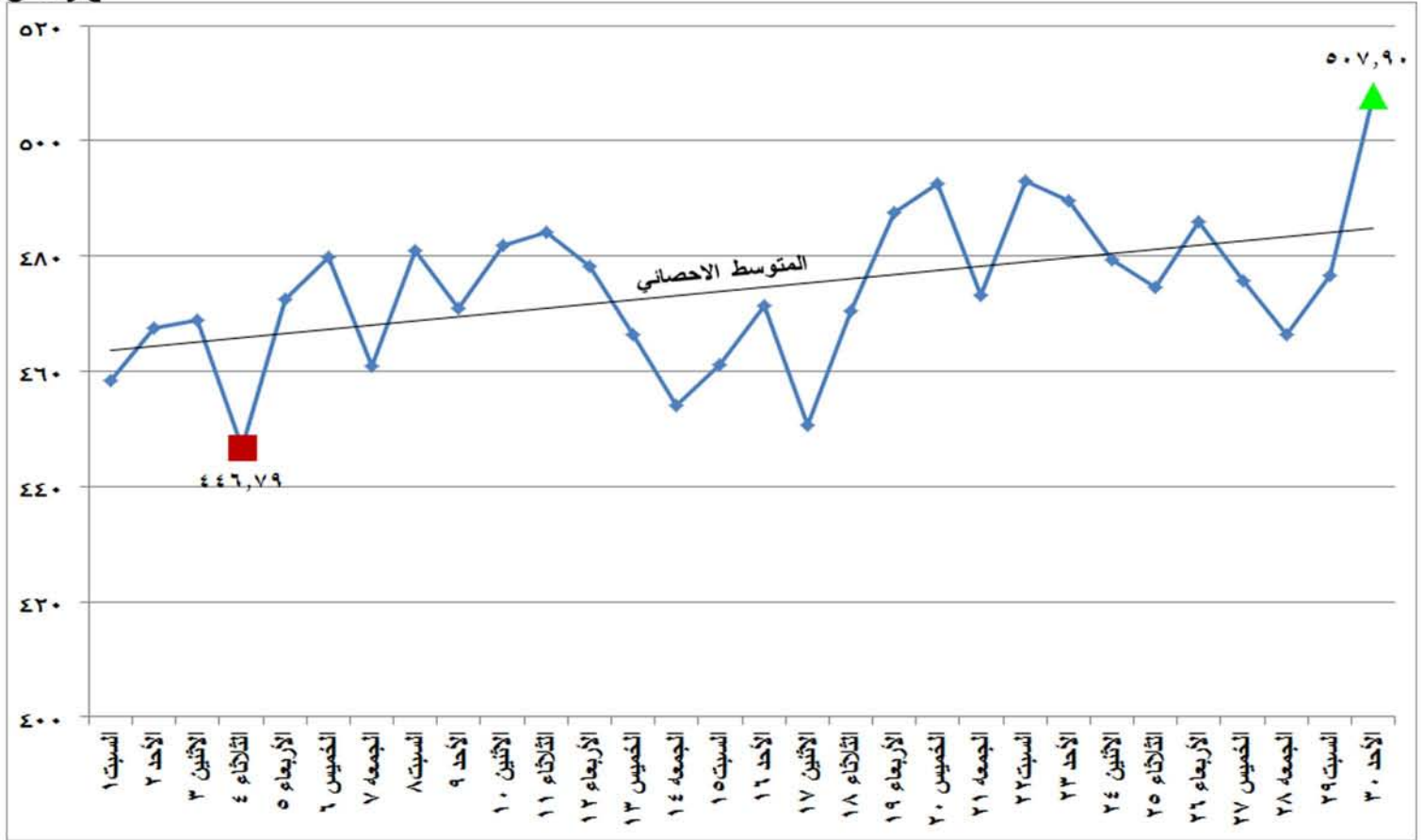
شكل (١٥) إجمالي الطاقة الكهربائية المنتجة من كل المصادر الأولية خلال شهر أبريل ٢٠١٦
