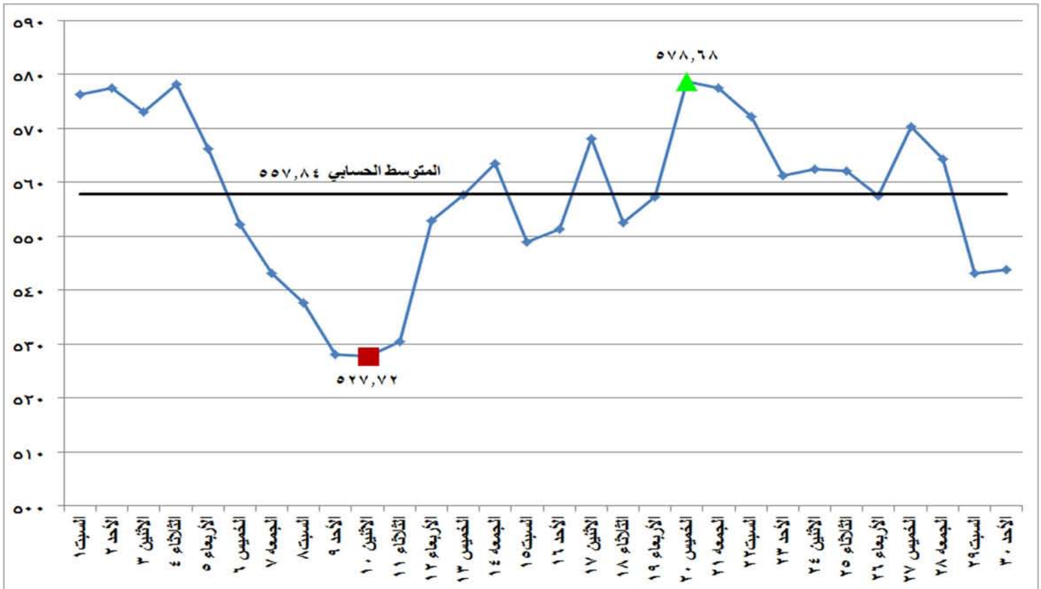
شكل (١٤) معامل انبعاثات غاز ثاني اكسيد الكربون المكافئ على مدى شهر أبريل ٢٠١٧
