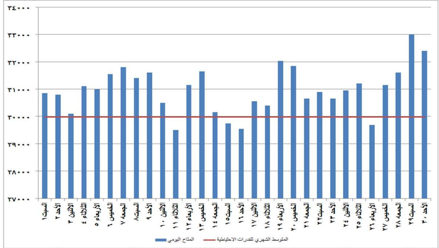
شكل (٢٧) القدرات المتاحة يوميا والمتوسط الشهري للقدرة الاحتياطية خلال شهر أبريل ٢٠١٧
