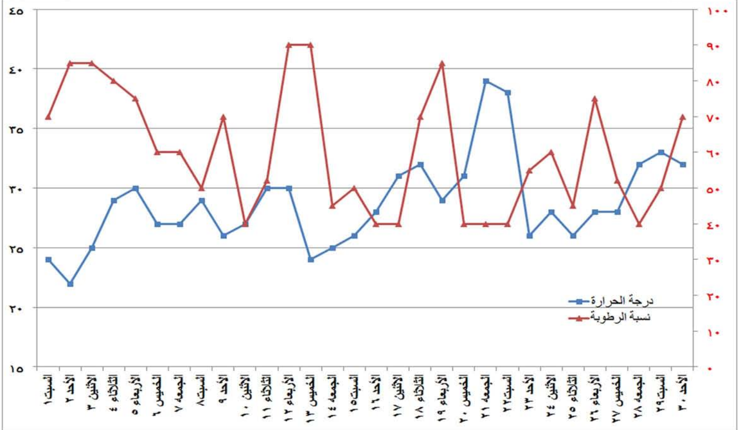
شكل (١١) التغيير في درجة الحرارة والرطوبة النسبية خلال شهر أبريل ٢٠١٧
