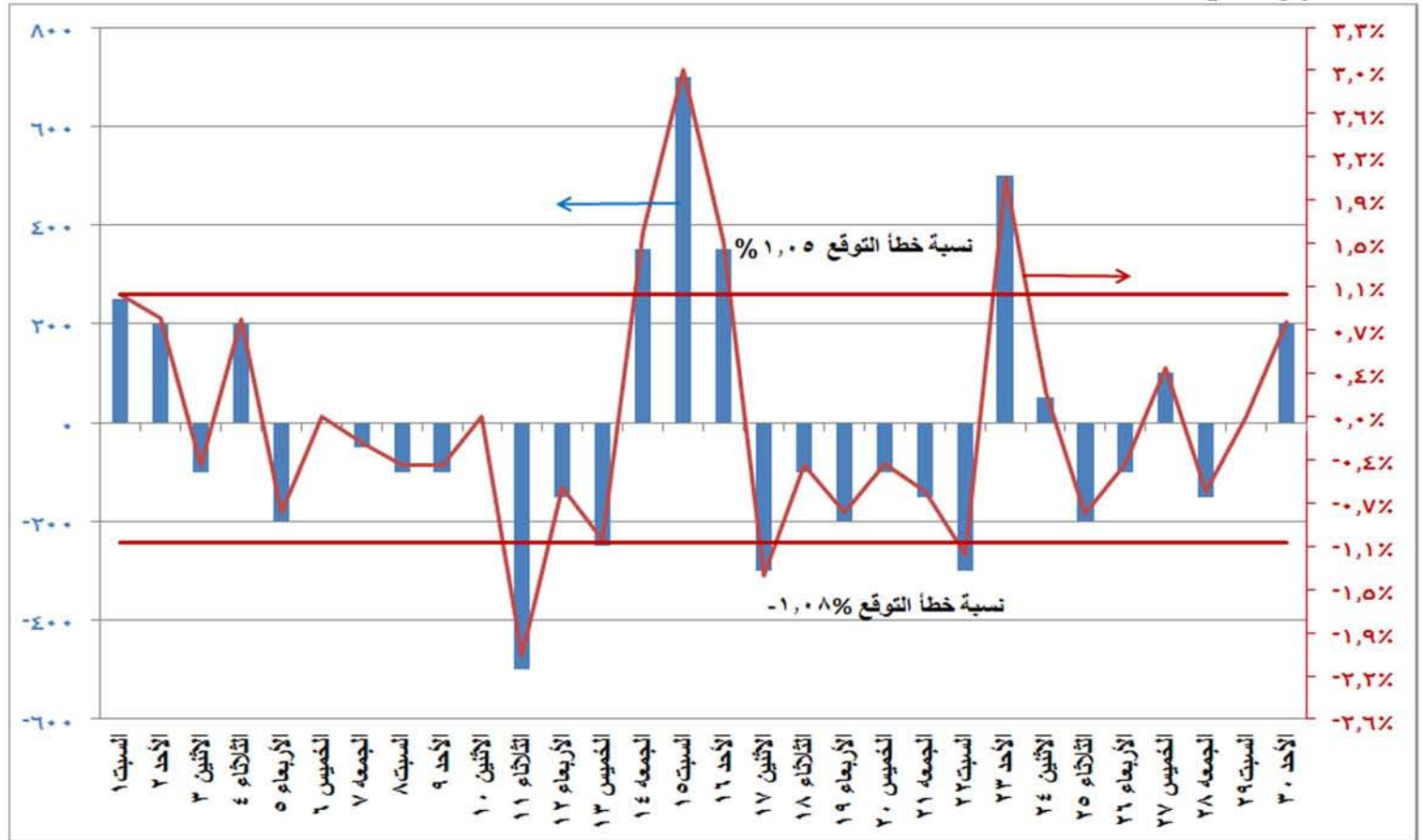
شكل (١٠) الفرق بين الحمل الأقصى المتوقع والمسجل فعليا ونسبة الفرق إلى الحمل المسجل فعليا خلال شهر أبريل ٢٠١٧
