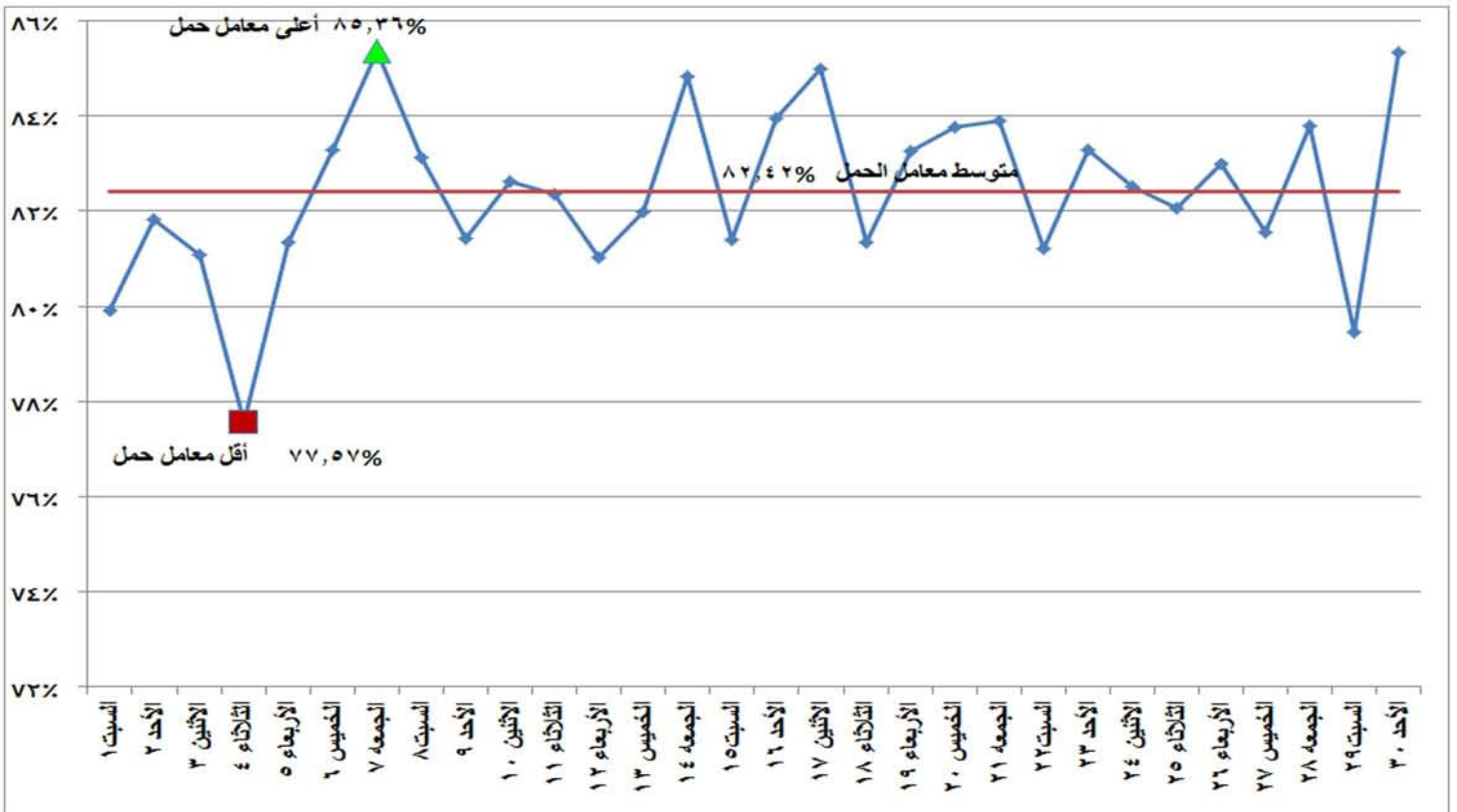
شكل (١٢) إجمالي معامل الحمل لوحدات الانتاج خلال شهر أبريل ٢٠١٧
