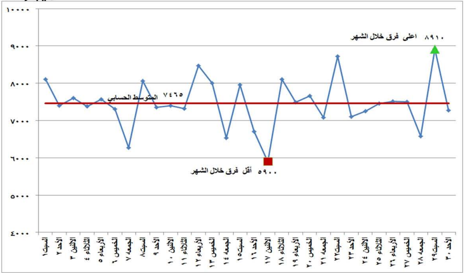
شكل (٣) الفرق بين أقصى وأدنى حمل خلال شهر أبريل ٢٠١٧
