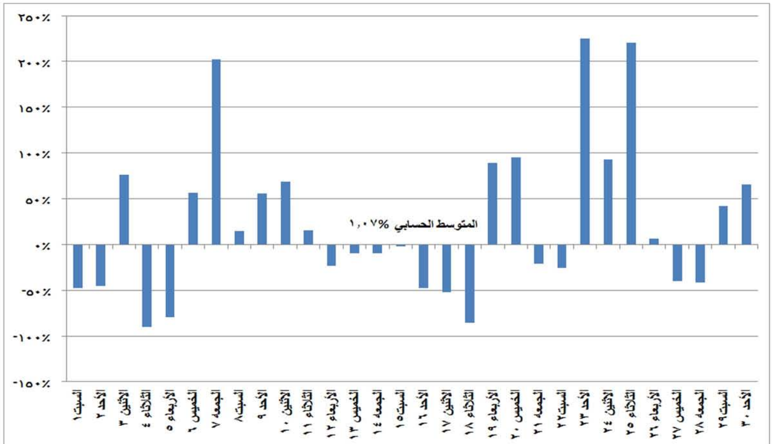
شكل (٢٦) نسب التغير في استخدام الرياح والشمس في إنتاج الطاقة الكهربائية خلال شهر أبريل ٢٠١٧ مقارنة بالشهر المماثل من العام السابق
