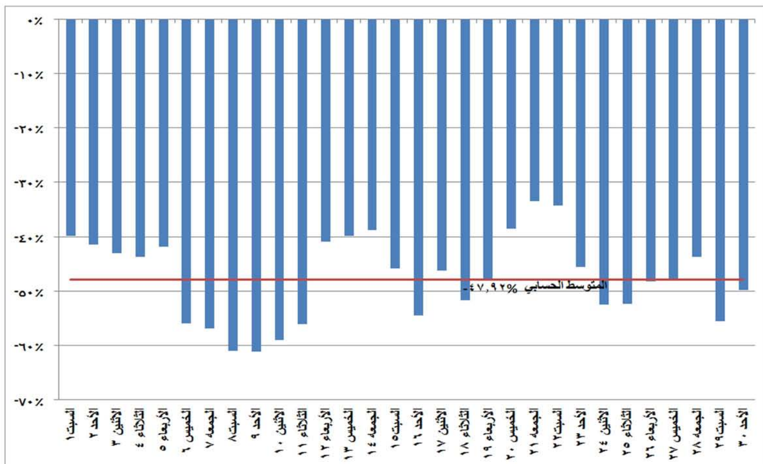
شكل (٢٠) نسب التغير في استخدام المازوت في إنتاج الطاقة الكهربائية خلال شهر أبريل ٢٠١٧ مقارنة بالشهر المماثل من العام السابق
